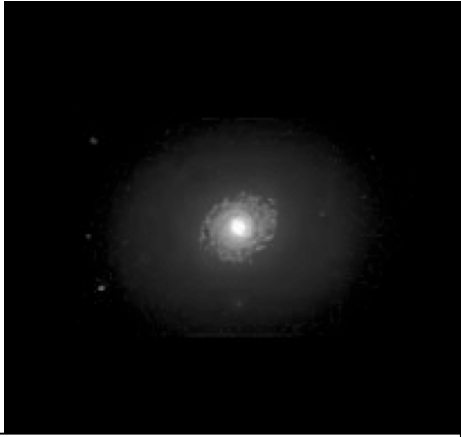
Visible - 1 (KPNO)
